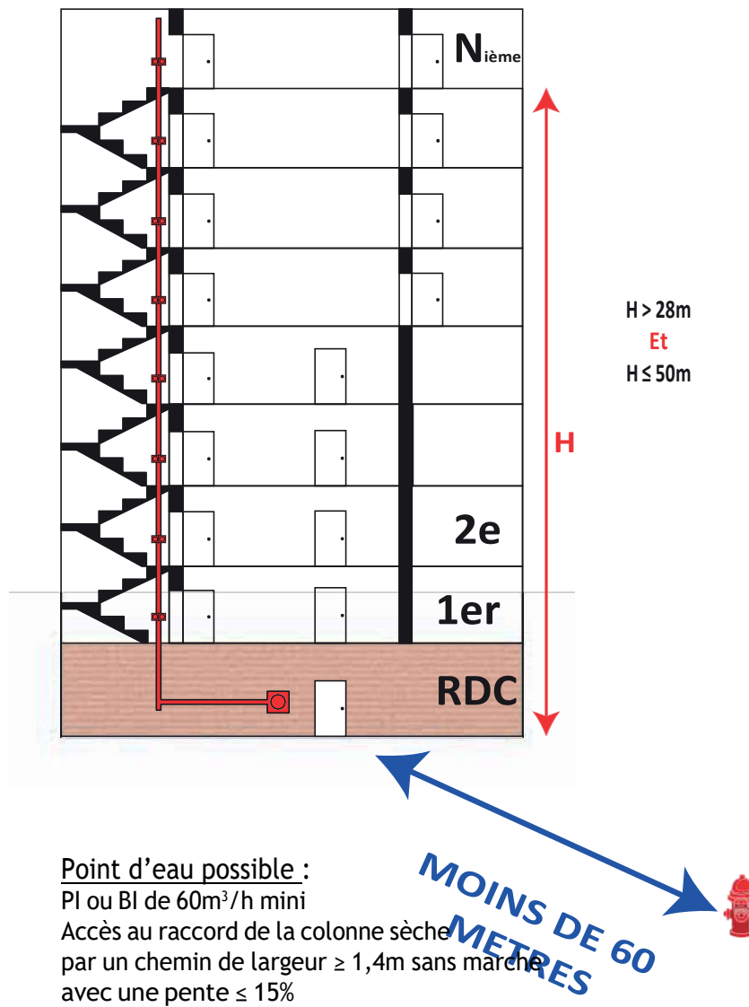
Figure 7 : Schéma de principe pour la couverture d'une habitation 4 ème famille avec colonne sèche imposée
