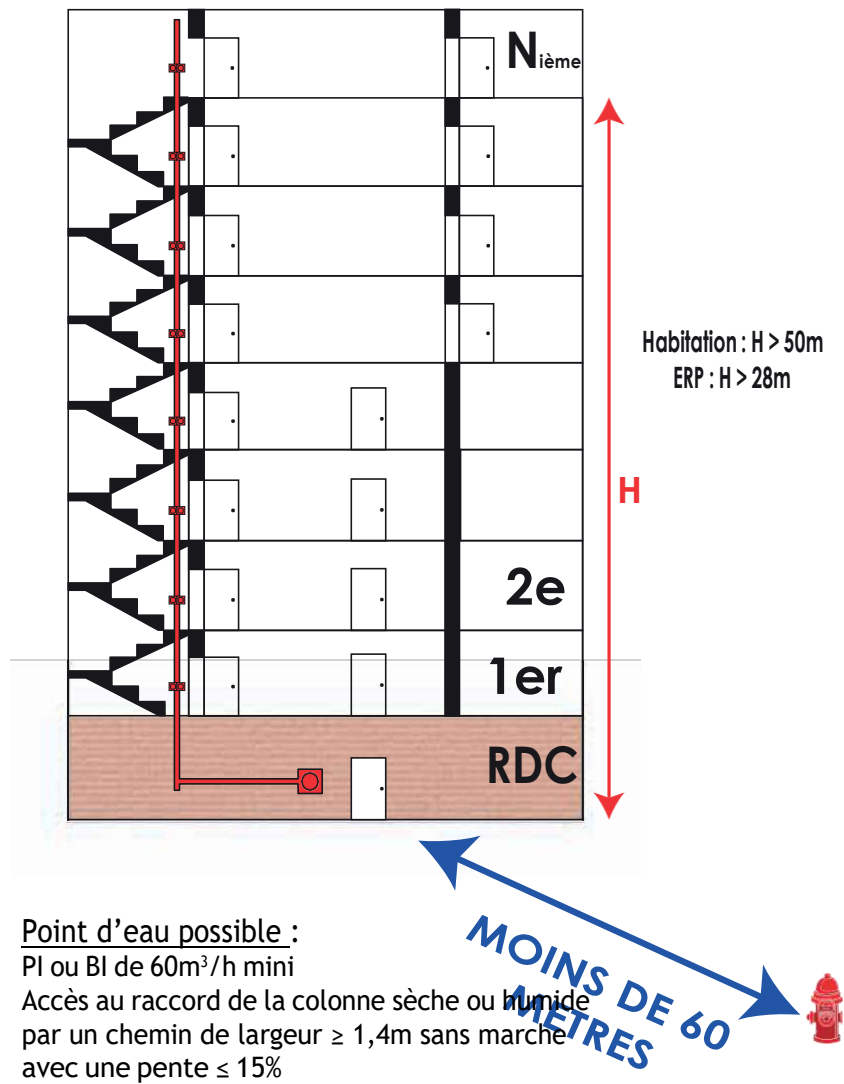
Figure 8 : Schéma de principe pour la couverture d'un IGH avec colonne sèche ou humide imposée
