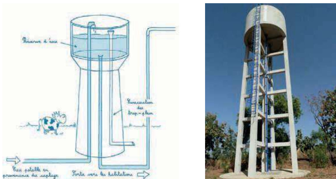
Figure 18 : Schéma de principe d'un château d'eau
